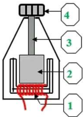
مكونات منوبة الدراجة
