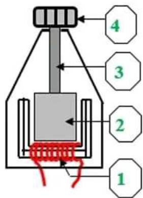
مكونات منوبة الدراجة
